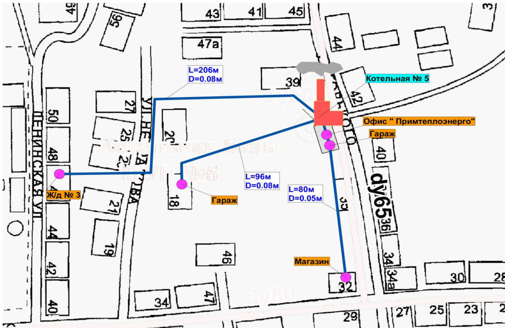
Рис. 2.5 – Схема теплоснабжения котельной №5 (с.Анучино)
