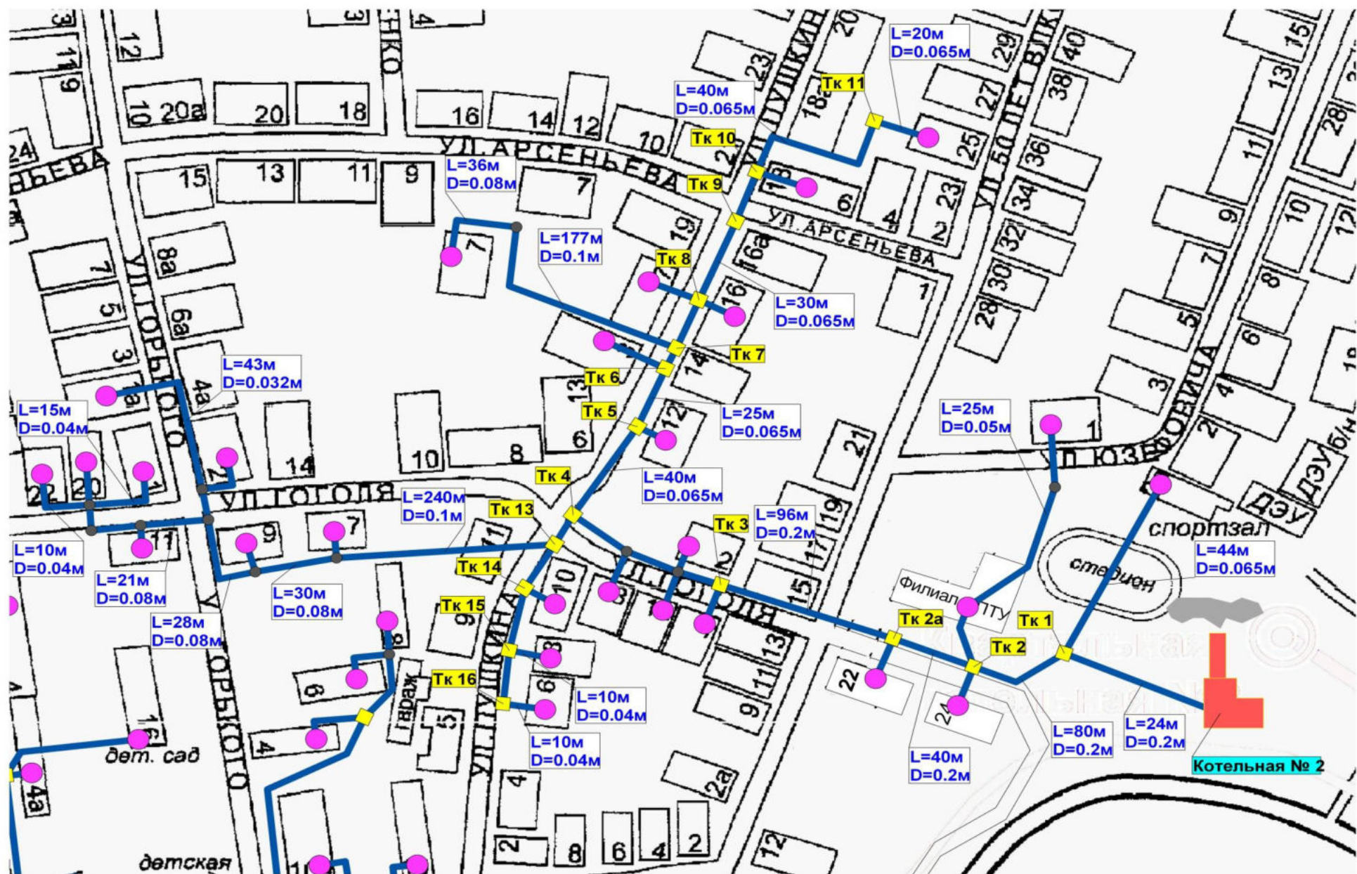
Рис. 2.4 – Схема теплоснабжения котельной №2 (с.Анучино)
