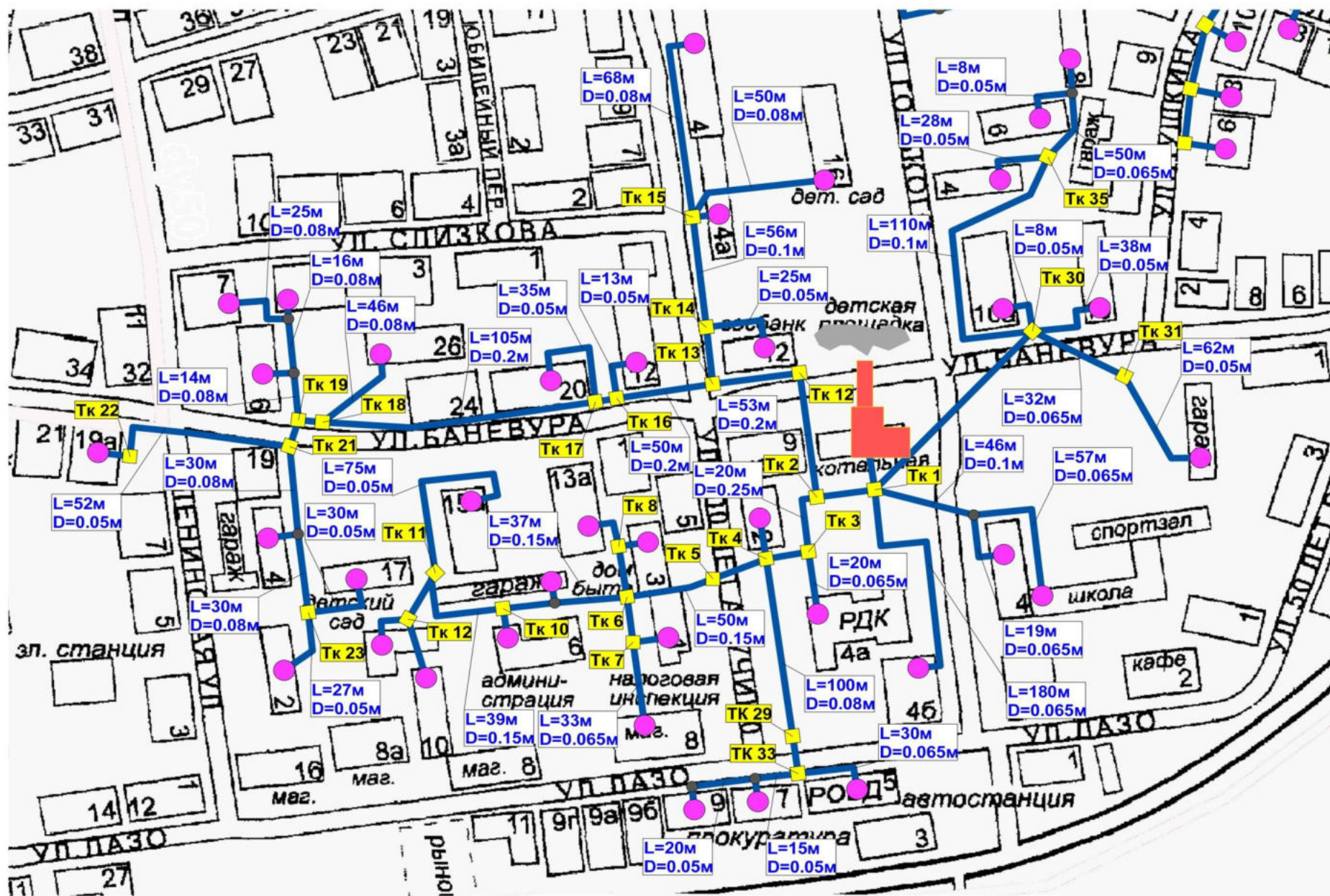
Рис. 2.3 – Схема теплоснабжения котельной №1(с.Анучино)
