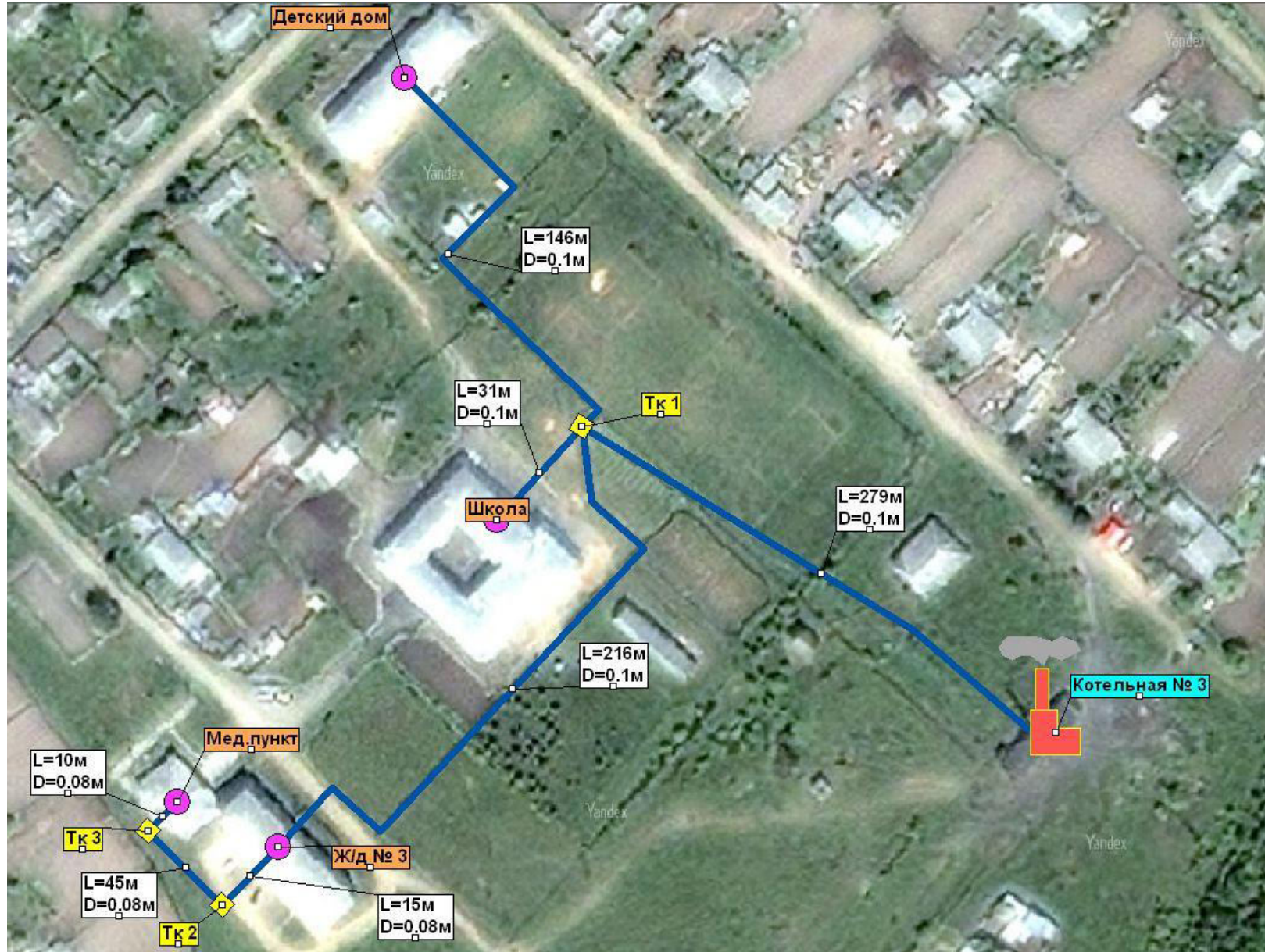
Рис. 2.7 – Схема теплоснабжения котельной №3(с.Новогордеевка)
