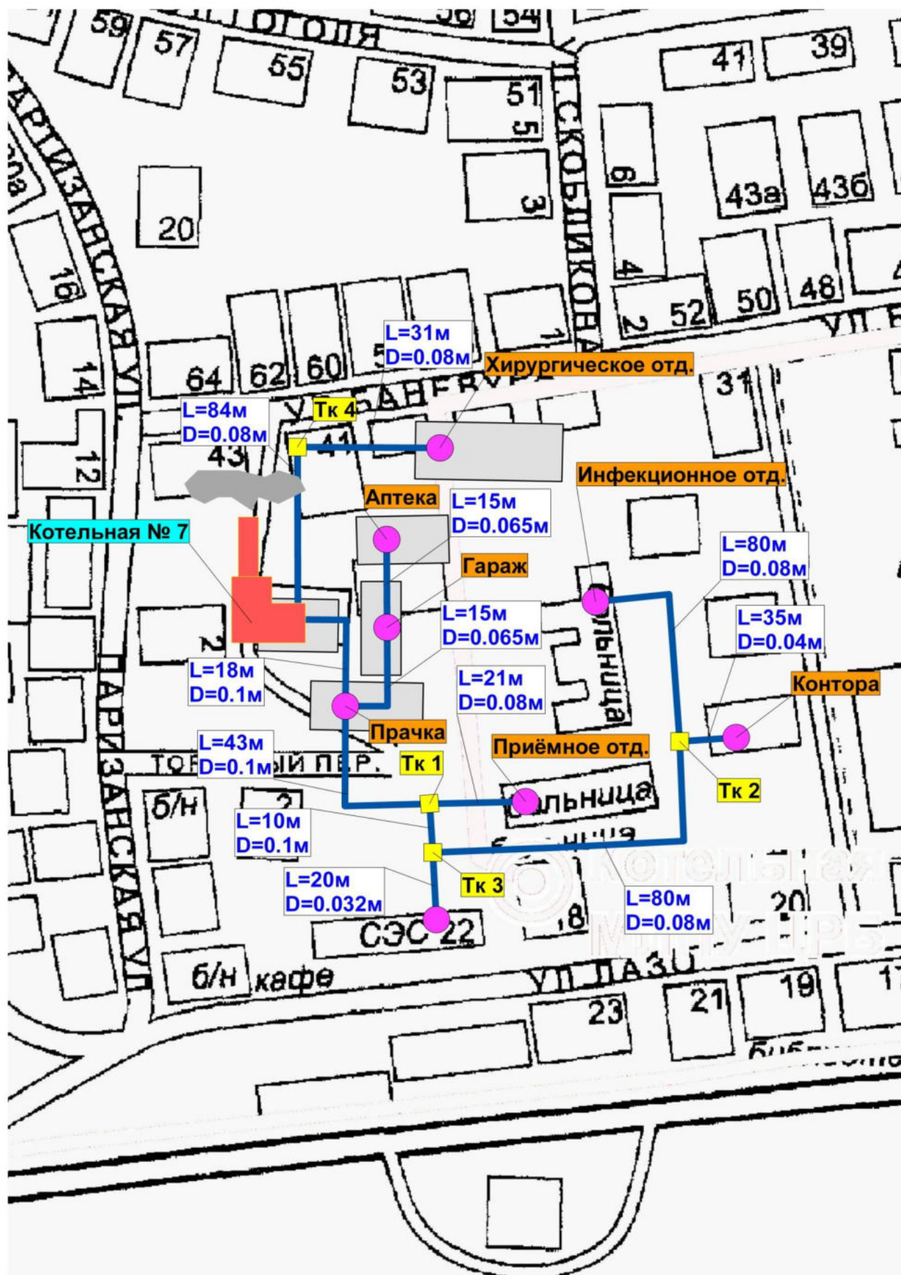
Рис. 2.6 – Схема теплоснабжения котельной №7(с.Анучино)
