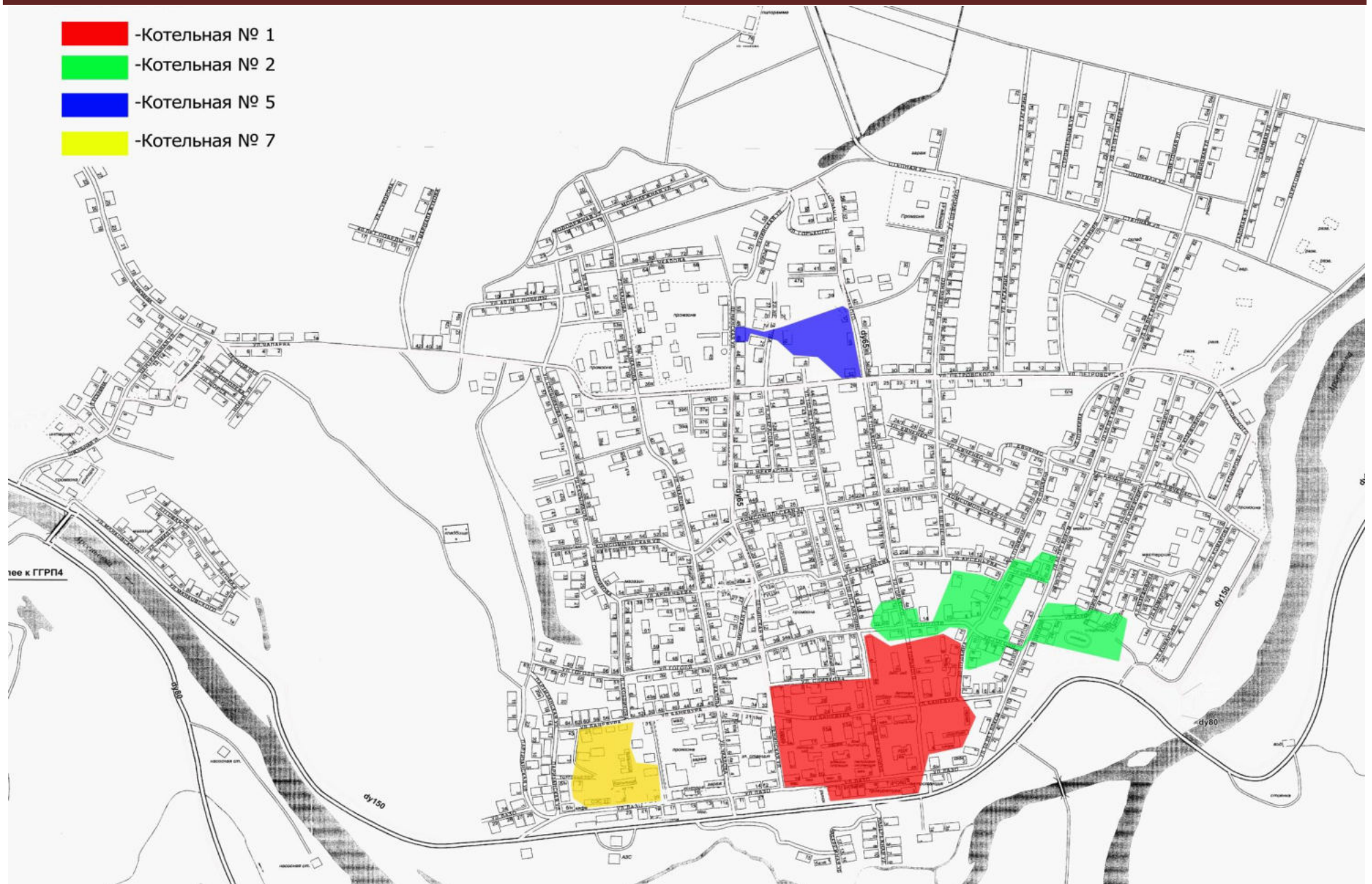
Рис. 2.1 – Зоны действия систем теплоснабжения сельского поселения Анучино
